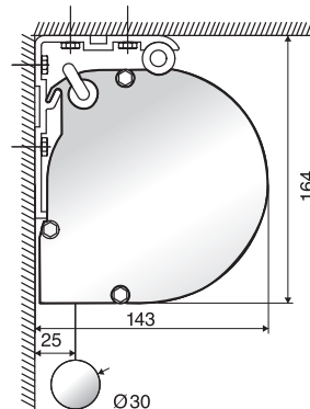
Verstelbare montagebeugels
